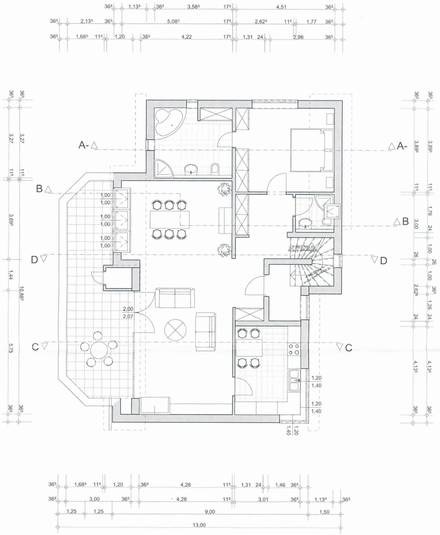
1. Obergeschoss
